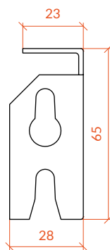
PERFIL
