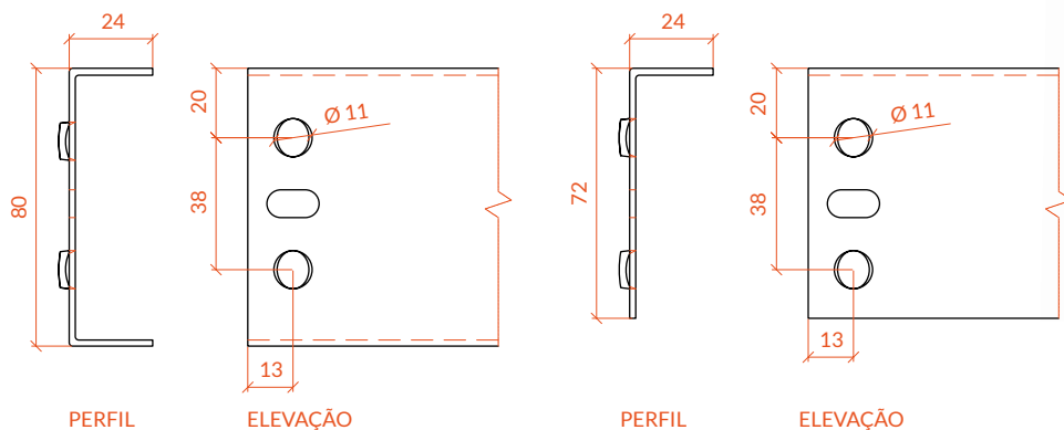
MONTANTES EM FORMA DE “U”
